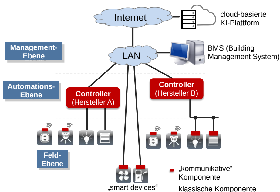
Abb. 2: Verbindung von Gebäudeautomation mit (cloud-basierter) AI-Plattform
